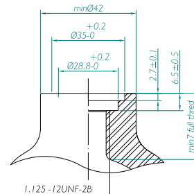
1.125-12UNF/ASME B 1.1
