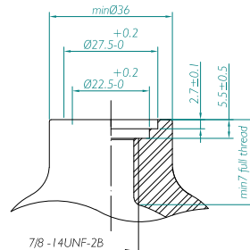
7/8-14UNF/ASME B 1.1
