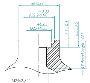
M25x2/ISO 15245-1
