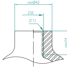
25E/ISO 11363-1
