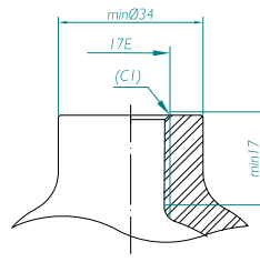
17E/ISO 11363-1
