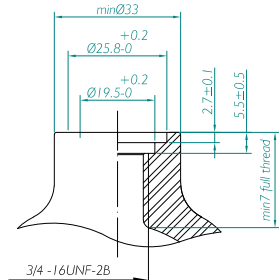
3/4-16UNF/ASME B 1.1
