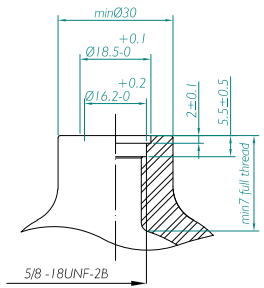
5/8-18UNF/ASME B 1.1
